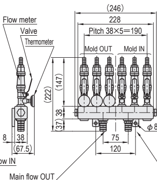
M-CMF-B-3-3
